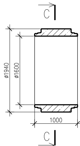
PRZEKRÓJ
